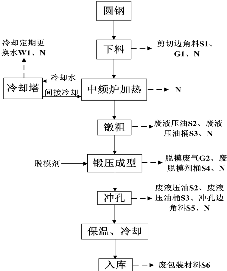
图 2-3 生产工艺流程及产污节点图
