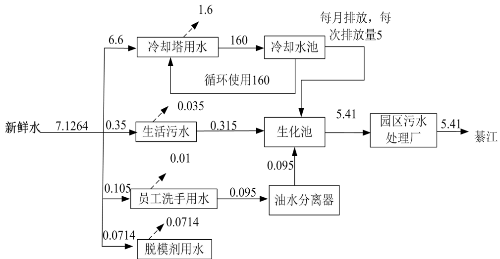
图 2-1 项目日最大用水、排水平衡图 单位：m 3 /d
