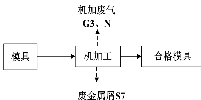
图2-4 模具维修工艺流程及产污环节图
