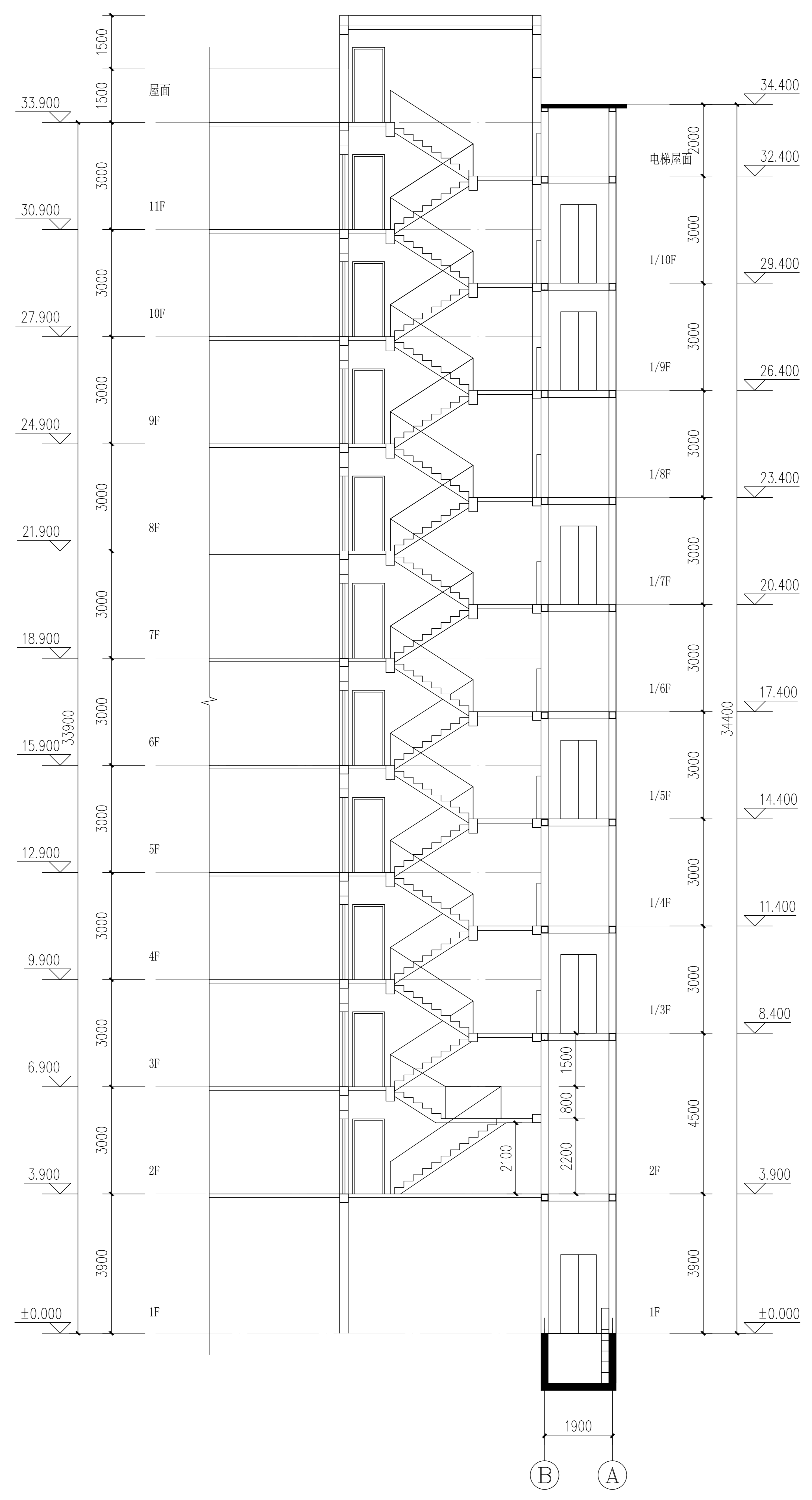
1-1剖面图 1:100
