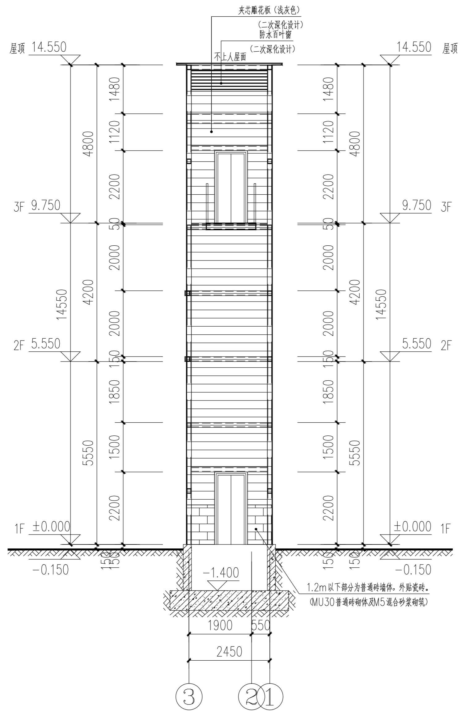
③—①轴立面图 1:100
