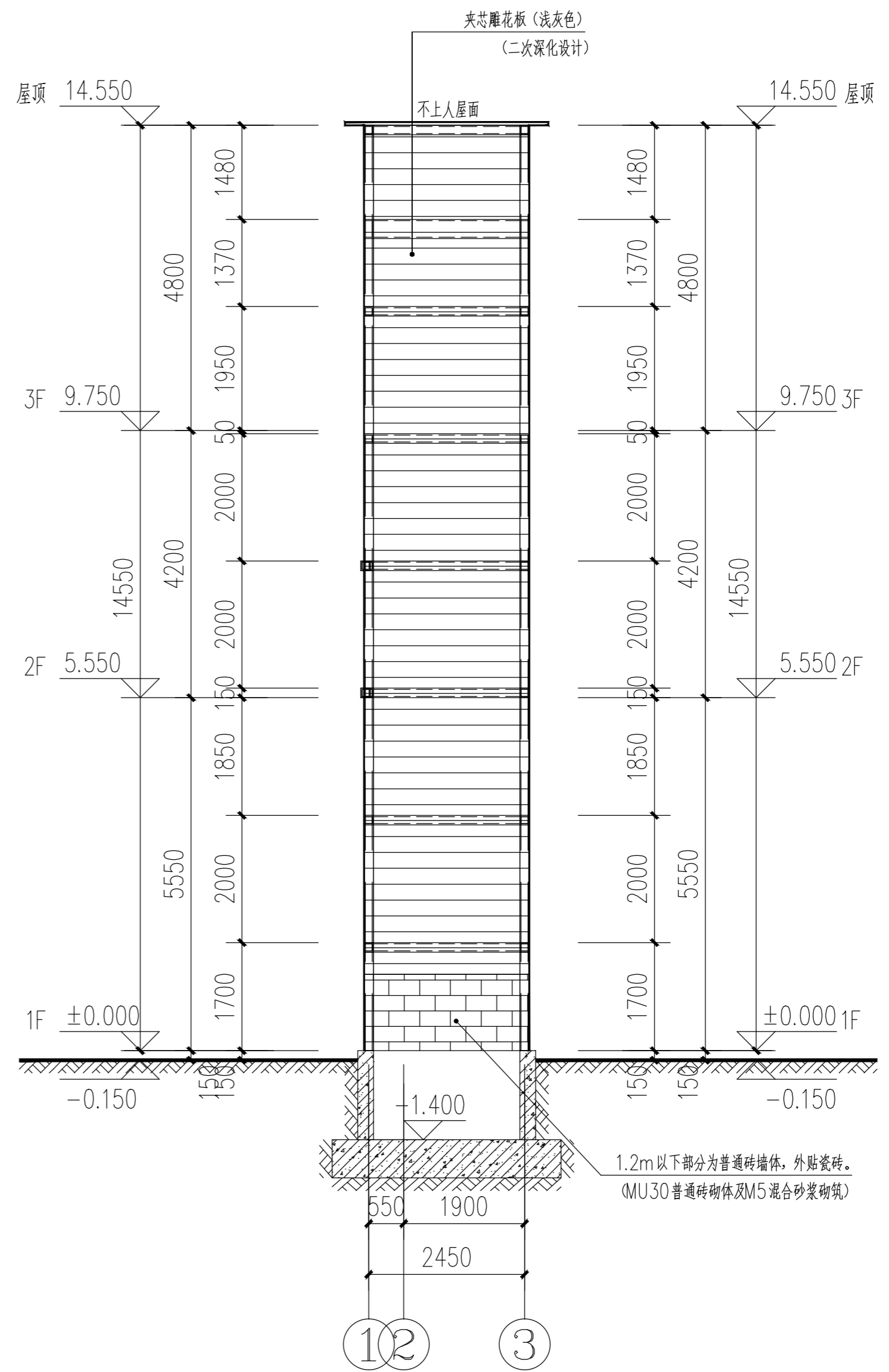
①—③轴立面图 1:100
