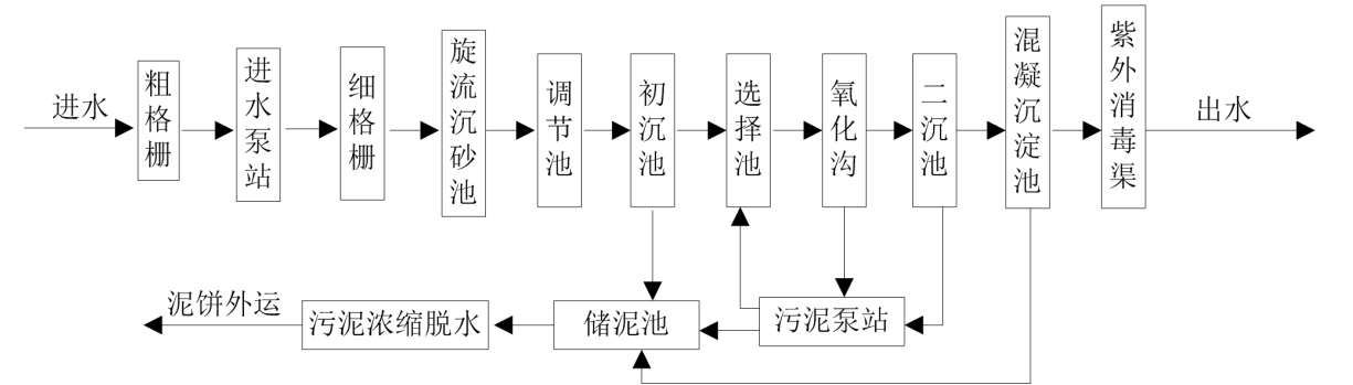
图 8.2-2 园区污水处理厂工艺流程图
