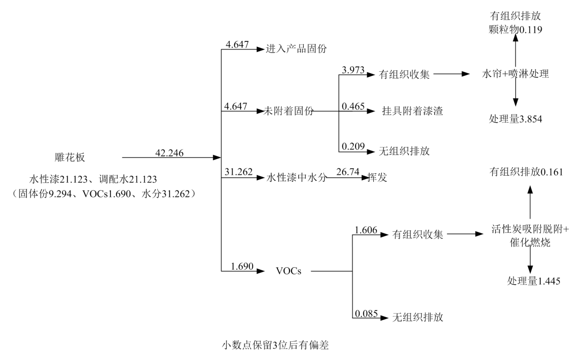
图 4.2-7 水性漆物料平衡图（t/a）
