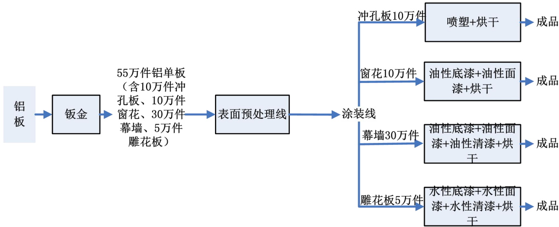
图 4.2-1 拟建项目总体工艺流程图
