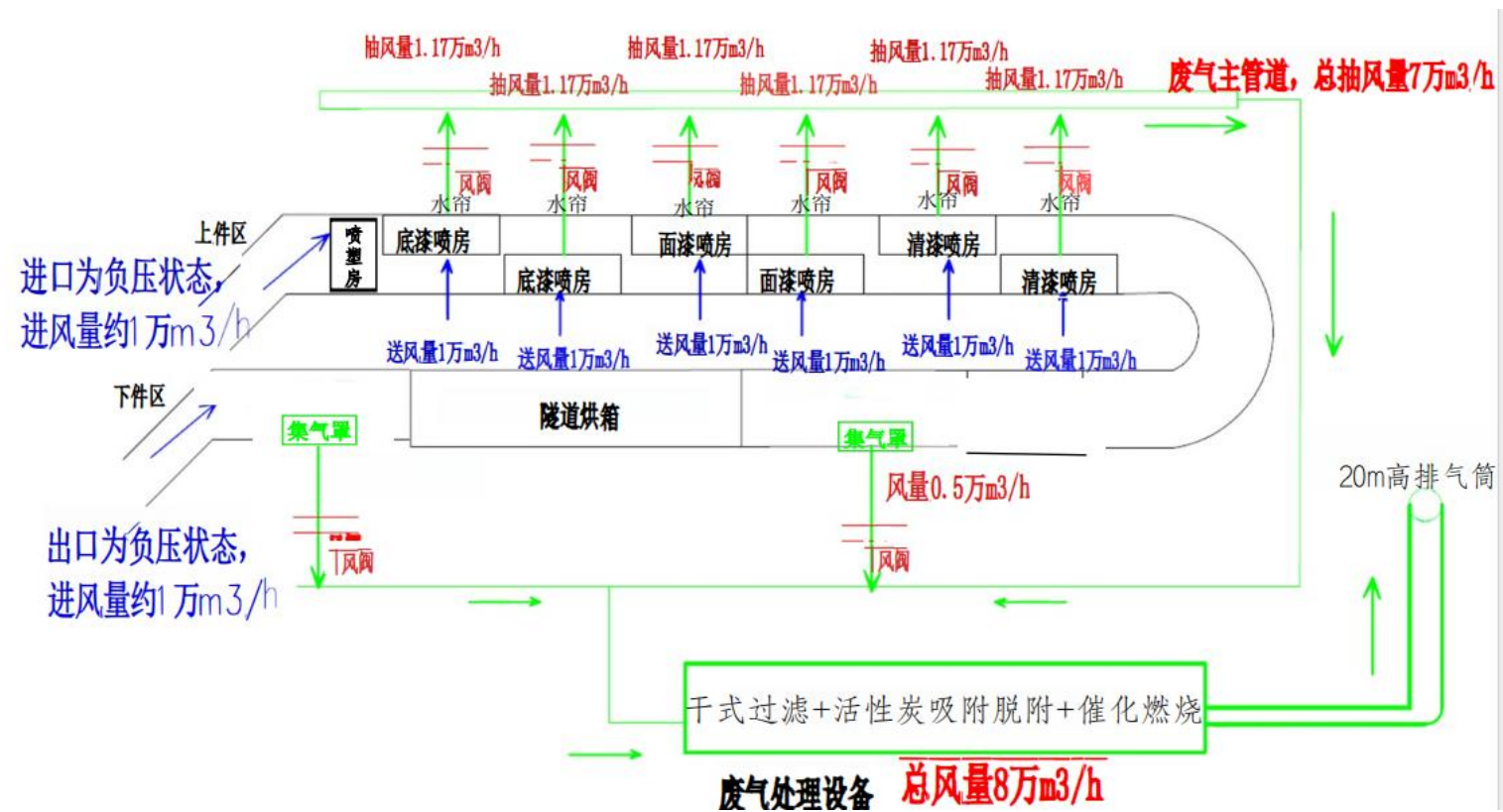
图 8.1-1 风平衡图 (6 个喷漆室同时运行时), 总风量控制在 8 万 m³/h
