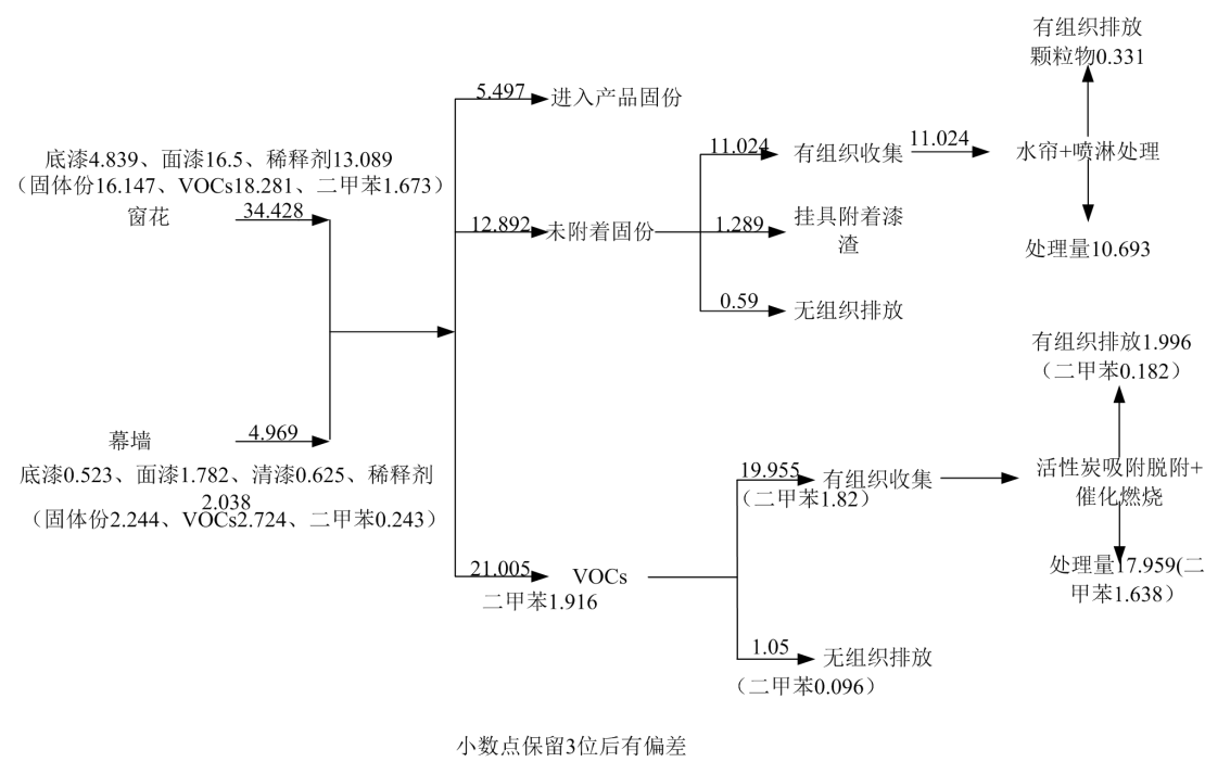
图 4.2-6 油性漆物料平衡图（t/a）
