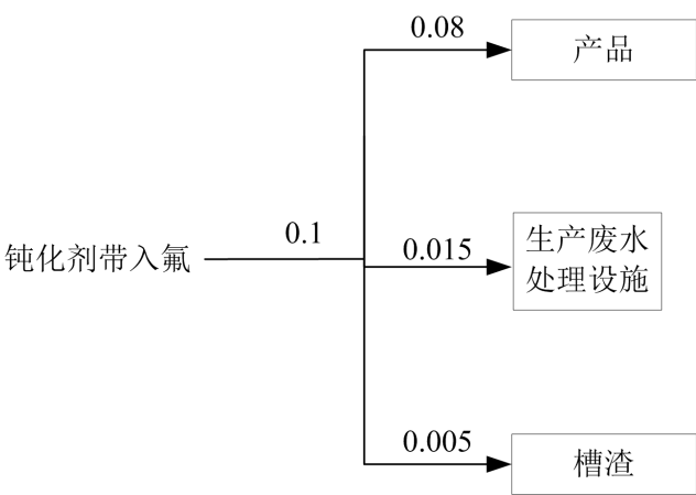
图 4.2-9 氟平衡图
