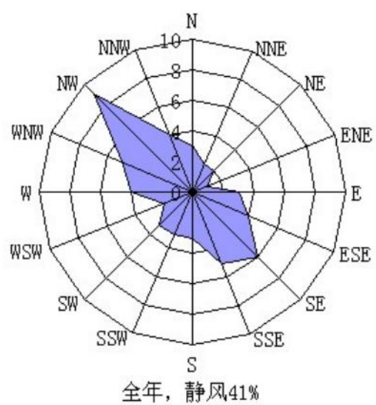
图 6.2-1 綦江区风频玫瑰图
