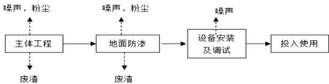
图 4.1-1 施工期产排污环节图
