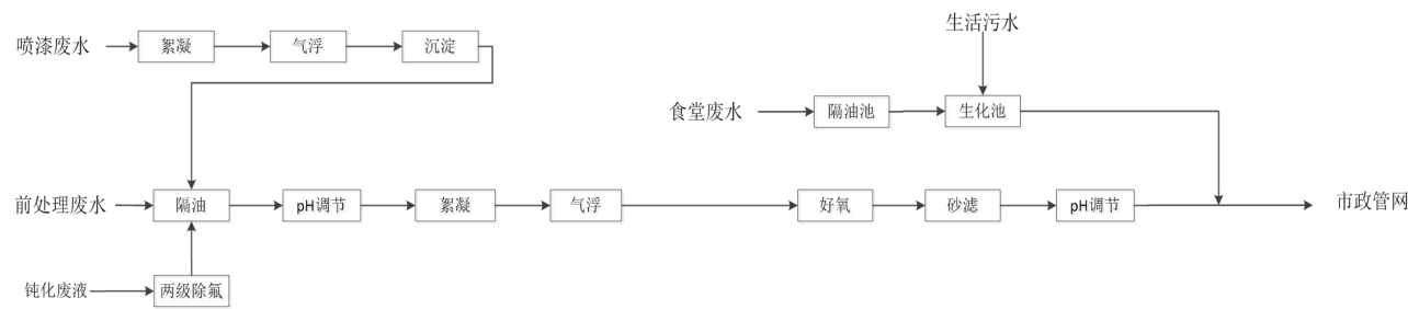
图 8.2-1 废水处理工艺流程图
