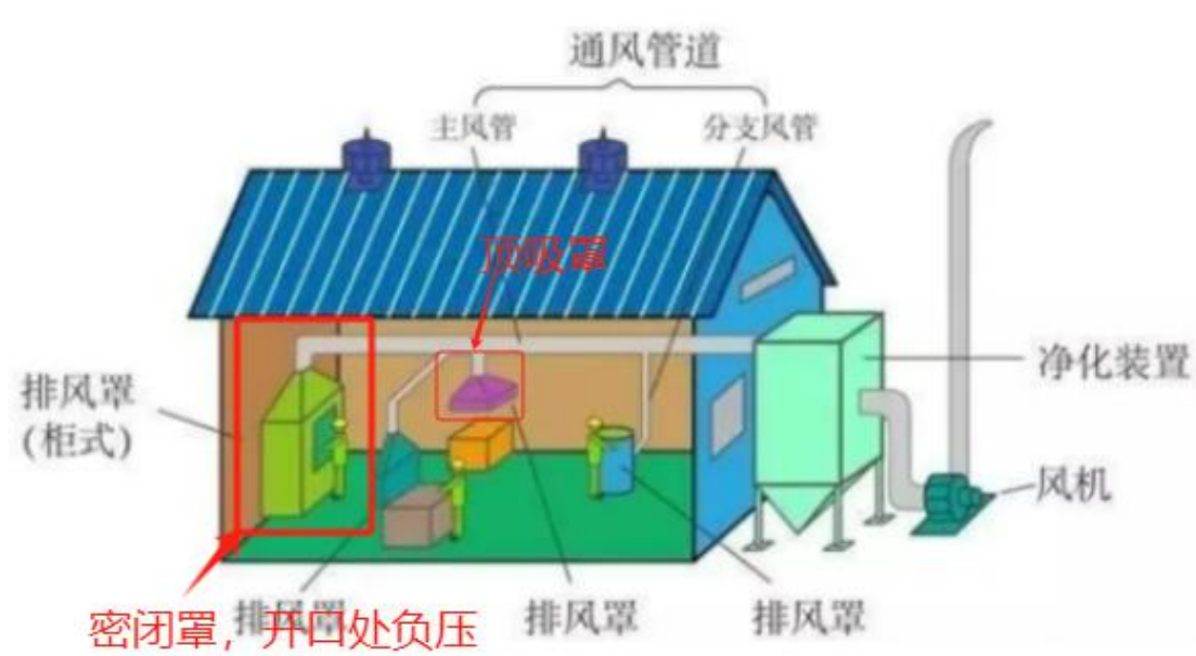
图 8.1-4 集气罩样图
