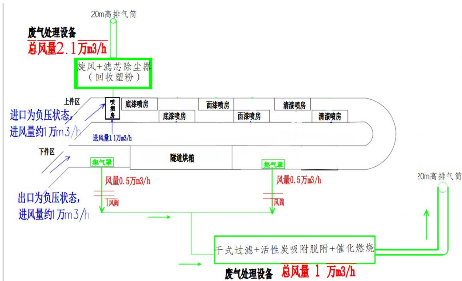
图 8.1-3 风平衡图（喷塑时），喷塑粉尘风量控制在 2.1 万 \text{m}^3/\text{h} ，喷塑烘干风量控制在 1 万 \text{m}^3/\text{h}
